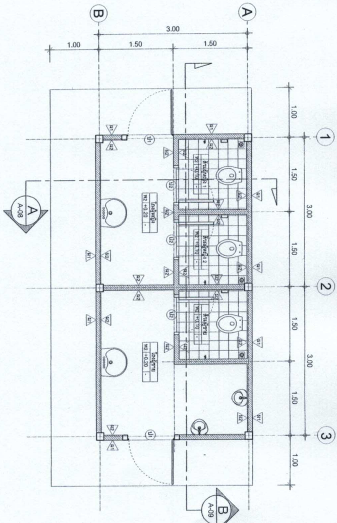
แปลนพื้น SCALE 1:50
