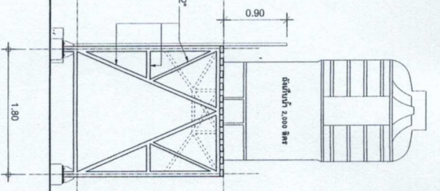
รูปด้านหลัง SCALE 1:50
