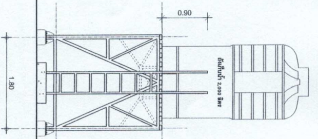
รูปด้านหน้า SCALE 1:50
