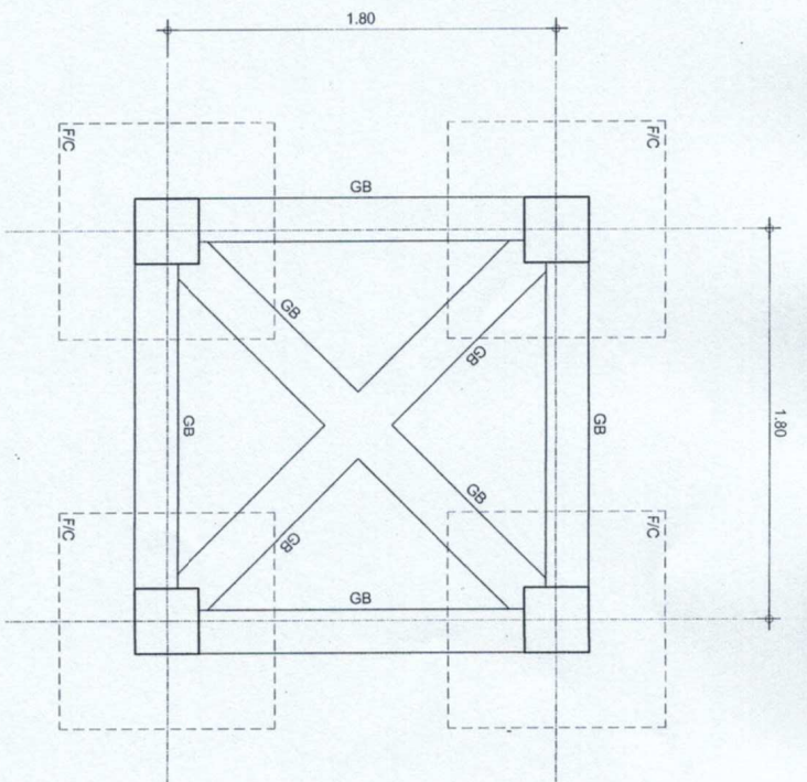
แปลนฐานราก/คานคอดิน SCALE 1:25
