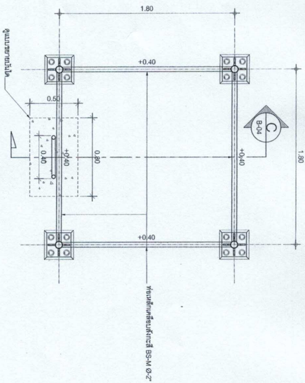
แปลนชั้นล่าง SCALE 1:25
