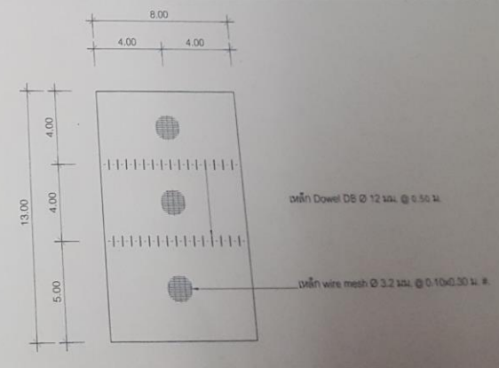
แปลนเหล็กเสริม ลาน คสล. หน้าเสาธง SCALE 1:200
