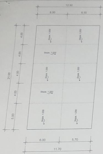
แปลนลาน คสล. หน้าอาคาร SCALE 1:200
