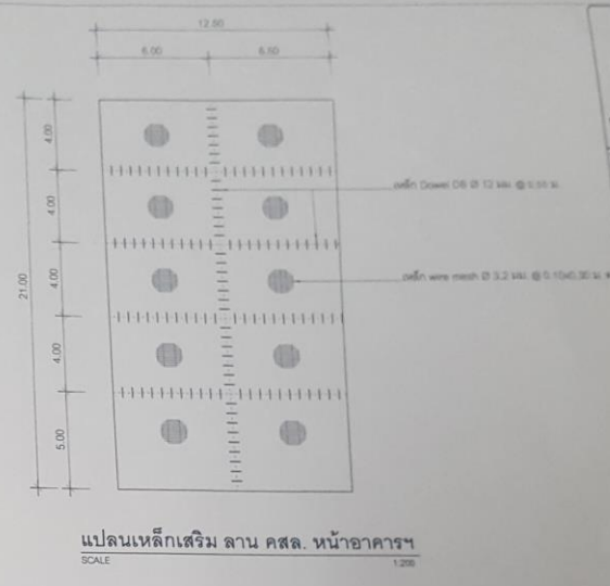
แปลนลาน คสล. หน้าอาคาร SCALE 1:200
